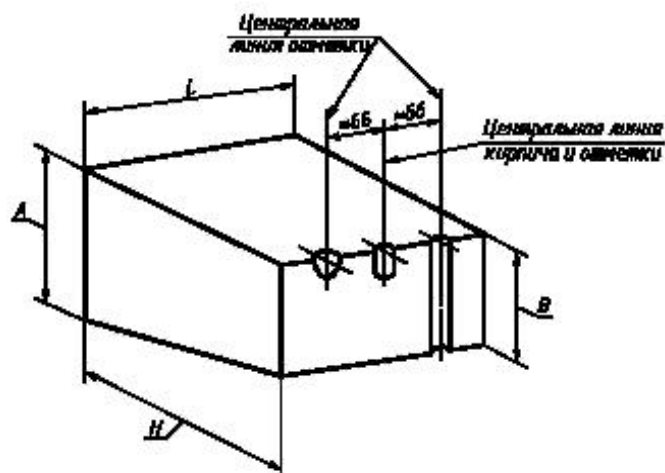
Рисунок В.1 — Расположение и типы выемок
